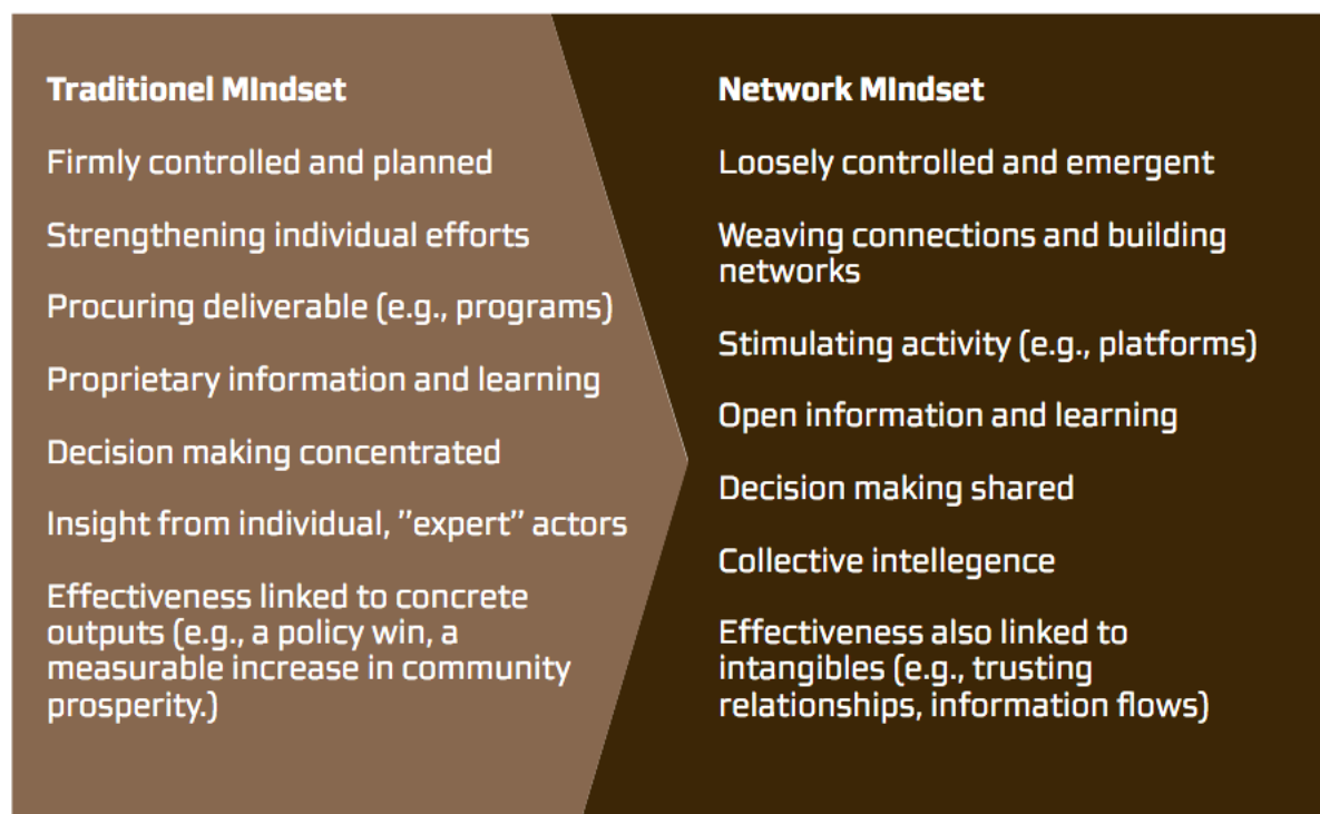
Figur 3, Netværksmodeller
